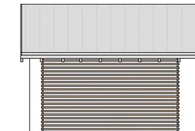
VISTA POSTERIORE
